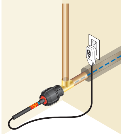
La faute de terre enfichable (GFC) modèle montré.
